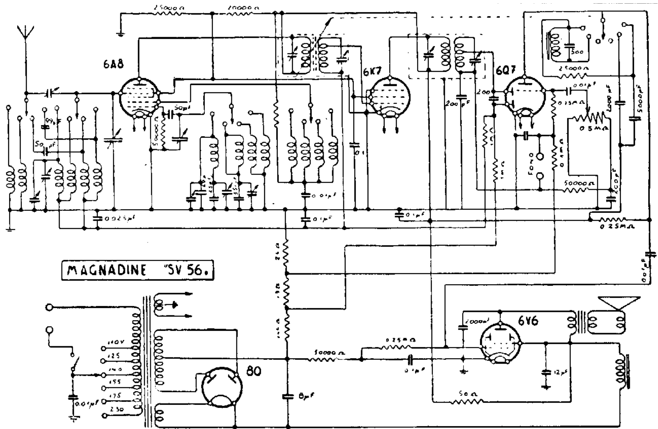
MAGNADINE RADIO — Mod. SV 56 e SV 56 c. — Produzione 1938-39. — Gamme: c. c. (13-25), c. (25-50), m. (200-550), l. (1000-2000) Media frequenza: 471 kHz.
